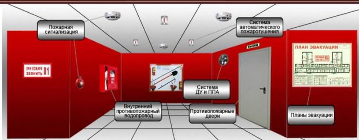
Рис. 2. Комплекс систем противопожарной защиты.
