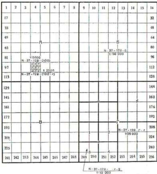
Рис. 44. Общая схема разграфки листа карты масштаба 1:100 000
