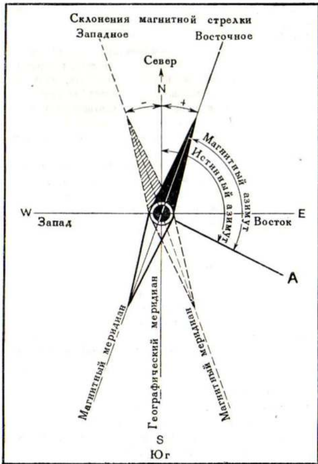
Рис. 47. Склонения магнитной стрелки и азимуты
