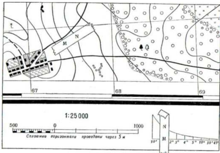
Рис. 45. Определение крутизн, ската по шкале заложений при помощи полоски бумаги
