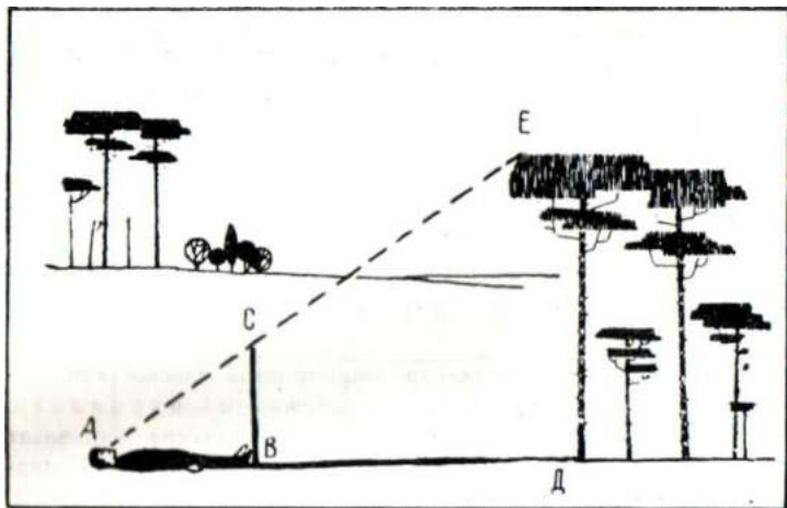
Рис. 39. Определение высоты предмета по своему росту
