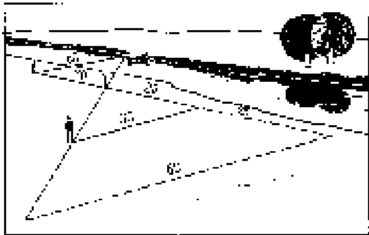
Рис. 36. Определение ширины реки шагами
