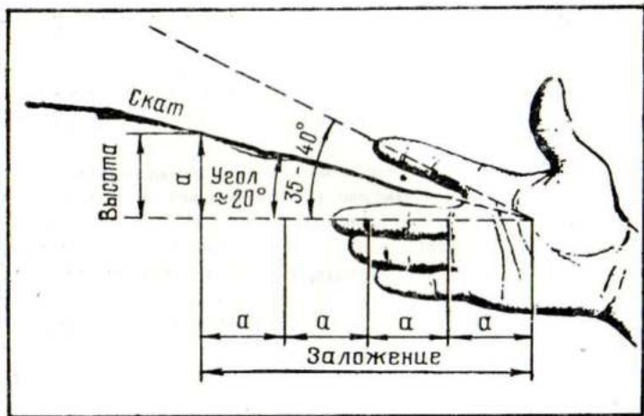
Рис. 46. определение крутизны ската на глаз
