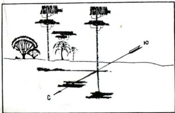
Рис. 67. Определение направления по тени
