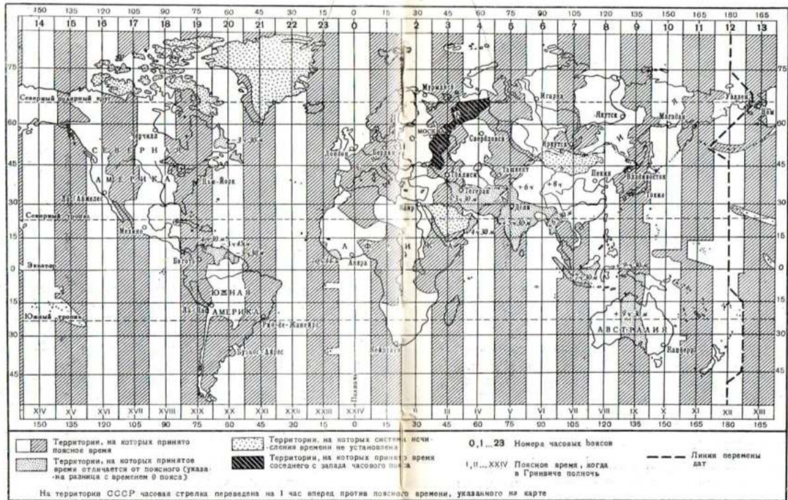
Рис. 54. Карта часовых поясов
