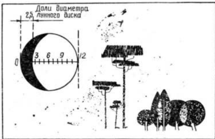
Рис. 58. Доли диаметра лунного диска
