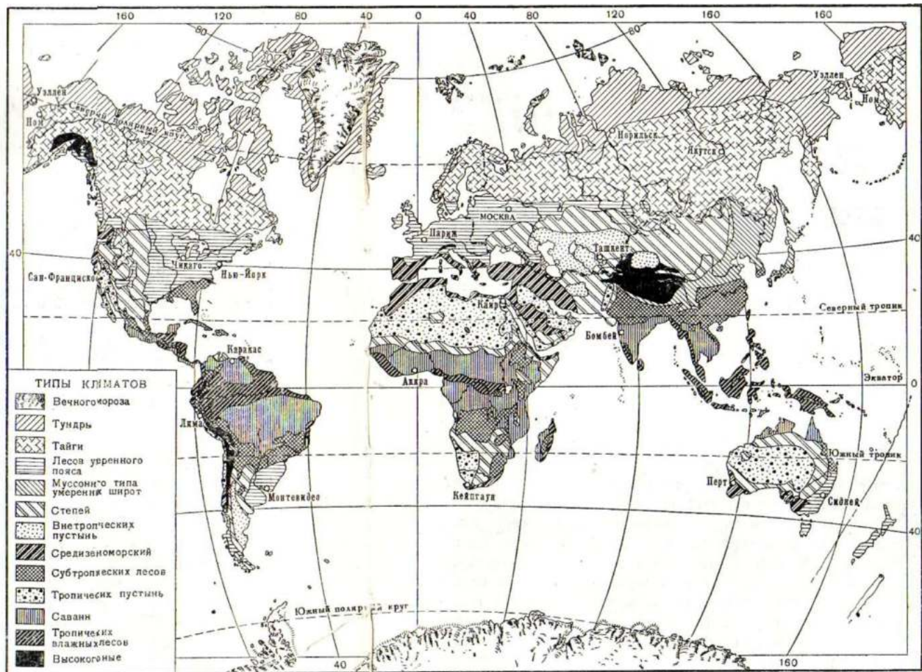
Рис. 3. Типы климатов земного шара (по Л. С. Бергу)
