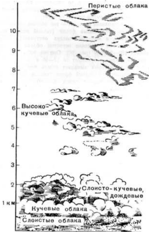
Рис. 90. Облака
