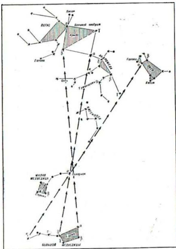
Рис. 71. Как найти созвездия Пегас, Андромеда и Овен?
