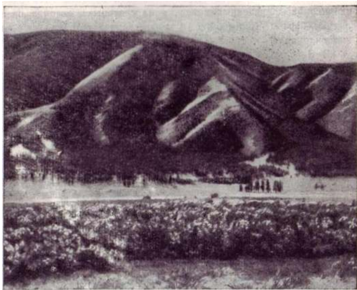
Рис. 72. Характер растительности в зависимости от экспозиции склонов
