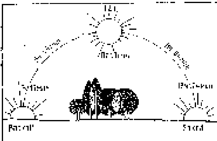
Рис. 48. Продолжительность дня и полдень по местному времени на широте 35° (12 марта)
