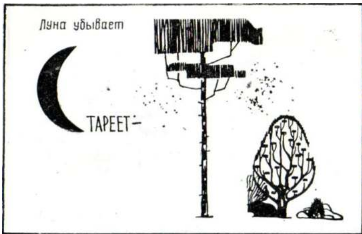
Рис. 60. Луна убывает
