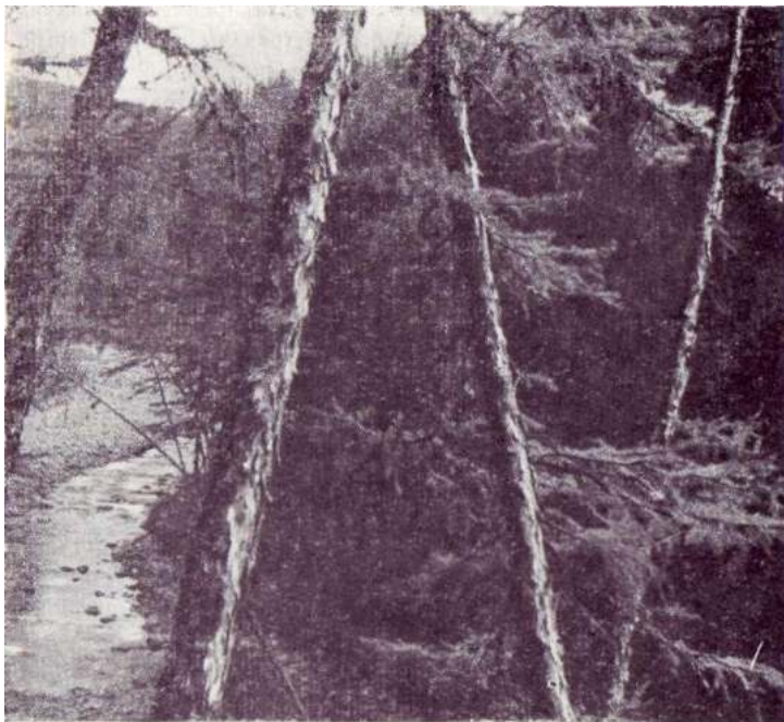
Рис. 8. Тайга. Южная Якутия
