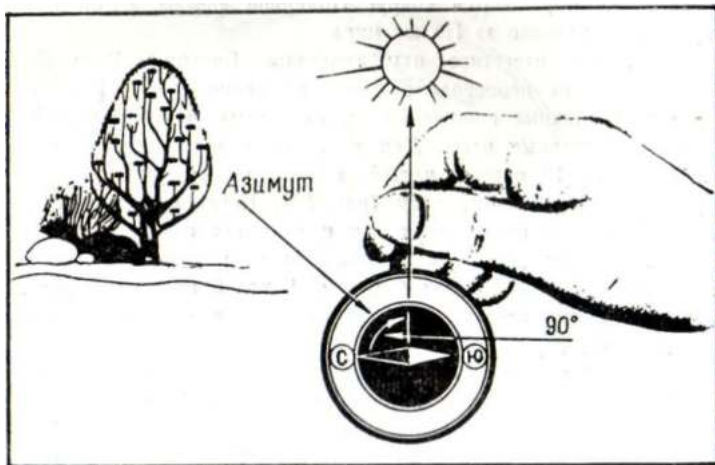
Рис. 56. Определение времени по Солнцу и компасу
