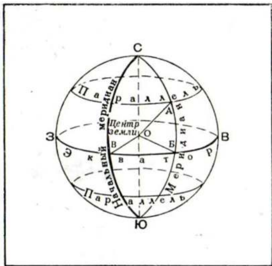
Рис. 40. Географические координаты
