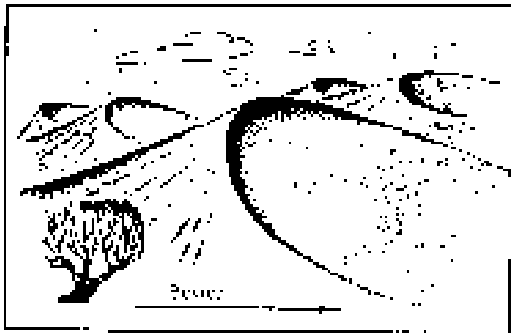
Рис. 75. Определение сторон горизонта по барханам
