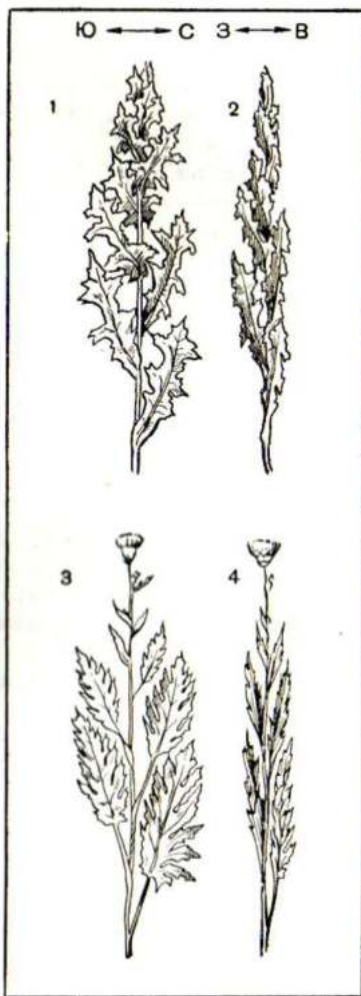
Рис. 82. Компасные растения — южноевропейское растение лактук и североамериканское растение силфиум:
