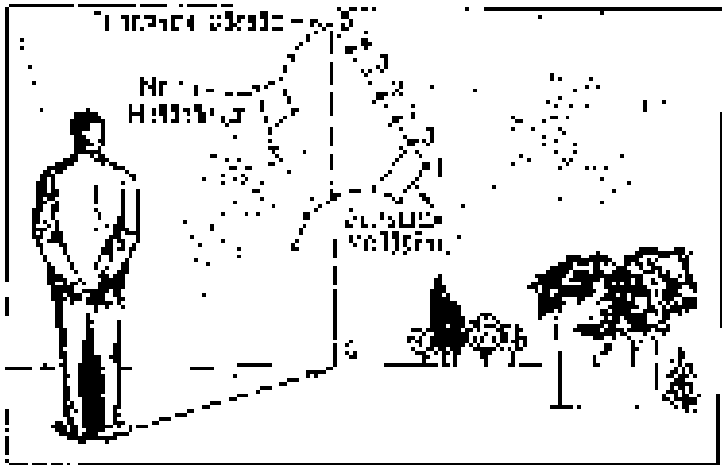
Рис. 51. Как найти Полярную звезду и взять направление на север
