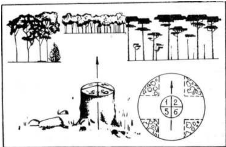
Рис. 73. Определение сторон горизонта по квартальному столбу на лесной просеке
