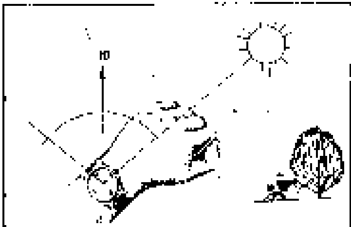
Рис. 66. Определение направления по Солнцу и часам после полудня
