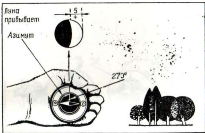
Рис. 61. Определение времени по компасу и Луне, когда она прибывает
