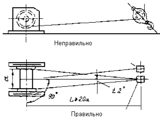
Рис. 4.2. Намотка каната на барабан
