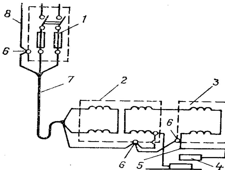
Рис. 7.1. Схема подключения сварочного трансформатора:
