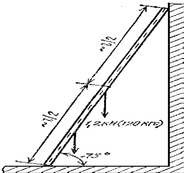
Рис. 5.5. Схема испытания приставной лестницы
