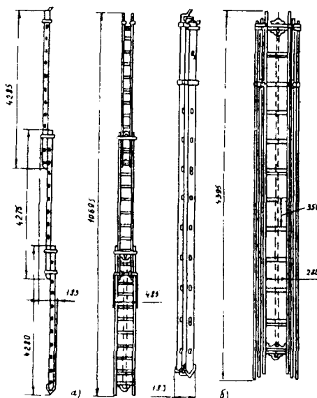
Рис. 5.1. Условное изображение приставной раздвижной лестницы Л-3К; а - рабочее положение; б - транспортное положение
