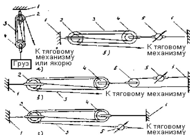
Рис. 4.4. Схема испытания многорольных блоков и полиспастов:
