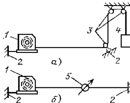
Рис. 4.1. Схема испытания лебедок
