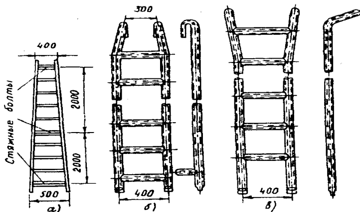
Рис. 5.2. Лестницы одноколенные:
